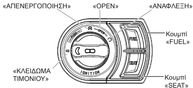
Κεντρικός διακόπτης
