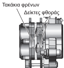
Εμπρόσθιο φρένο
