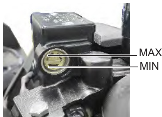
Παράθυρο ελέγχου υγρού φρένων
