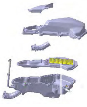
Στοιχείο φίλτρου
