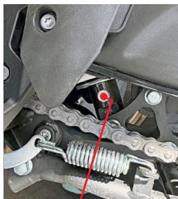
Ρυθμιστής (3) ταχύτητας επαναφοράς
