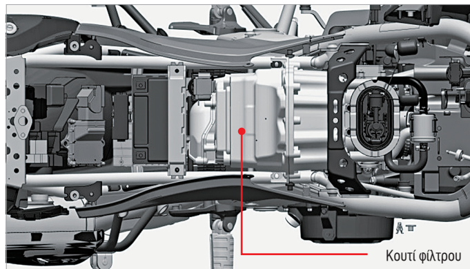
Φίλτρο αέρα
